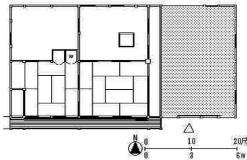
図 18 矢島寛家主屋復原平面図
