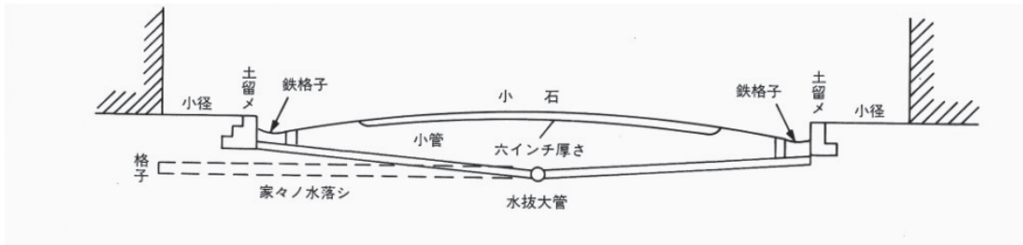
図10 プラントン「旧居留地道路溝渠之図」(『横浜下水道史』横浜市下水道局 1993年より)
